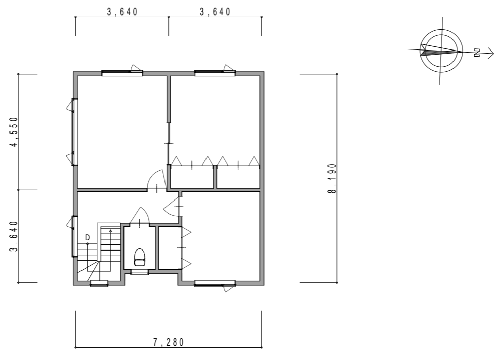
2階 平面図
