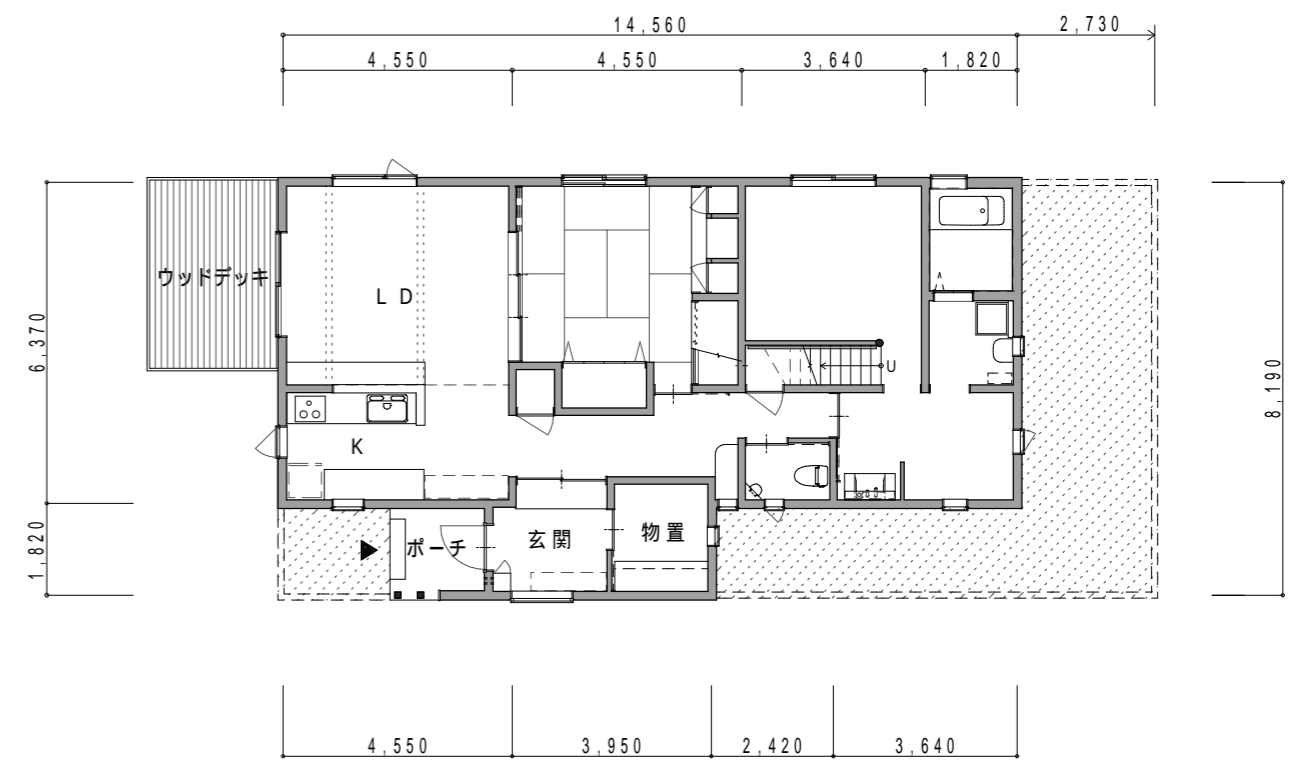
1階 平面図
